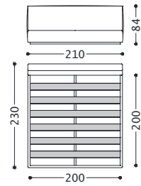
1DILLA200 2DILLA200
