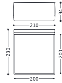
1DILLA200BH 2DILLA200BH
