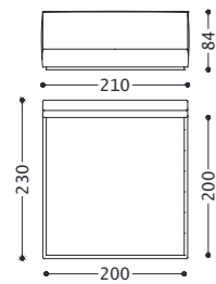
1DILLA200B 2DILLA200B
