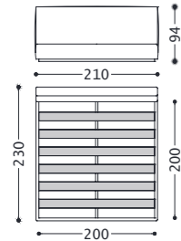
1DILLA200H 2DILLA200H
