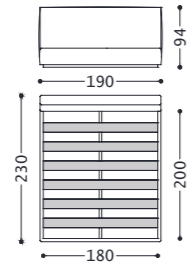
1DILLA180H 2DILLA180H
