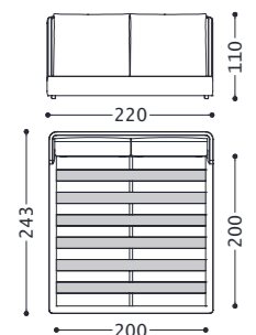
1NKLLA200H 2NKLLA200H
