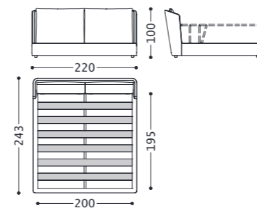
1NKLLA200AF 2NKLLA200AF
